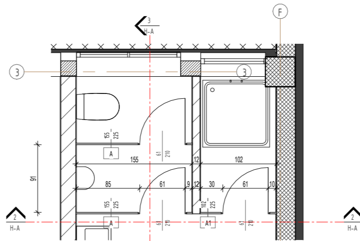
1 Tlocrt HPL A+A1 1:50
