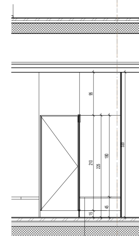
3 Presjek HPL D6-b 1:50
