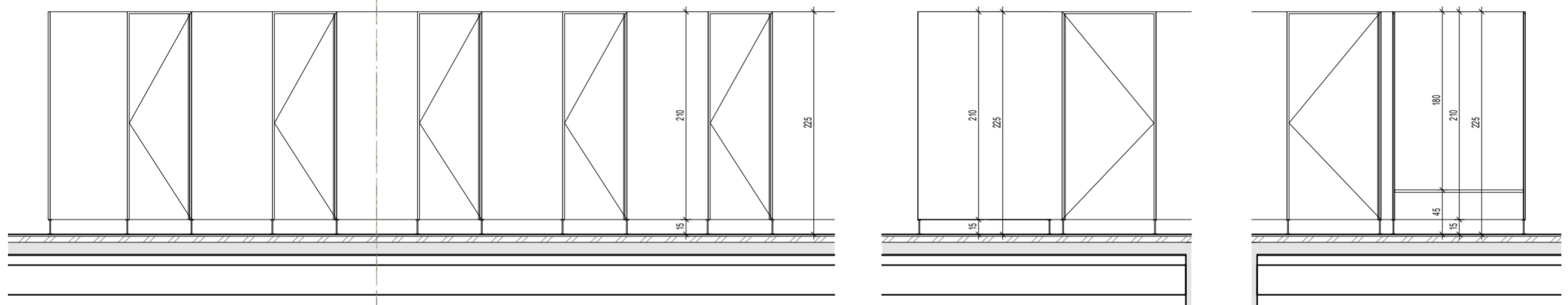
2 Presjek HPL D2-a 1:50
