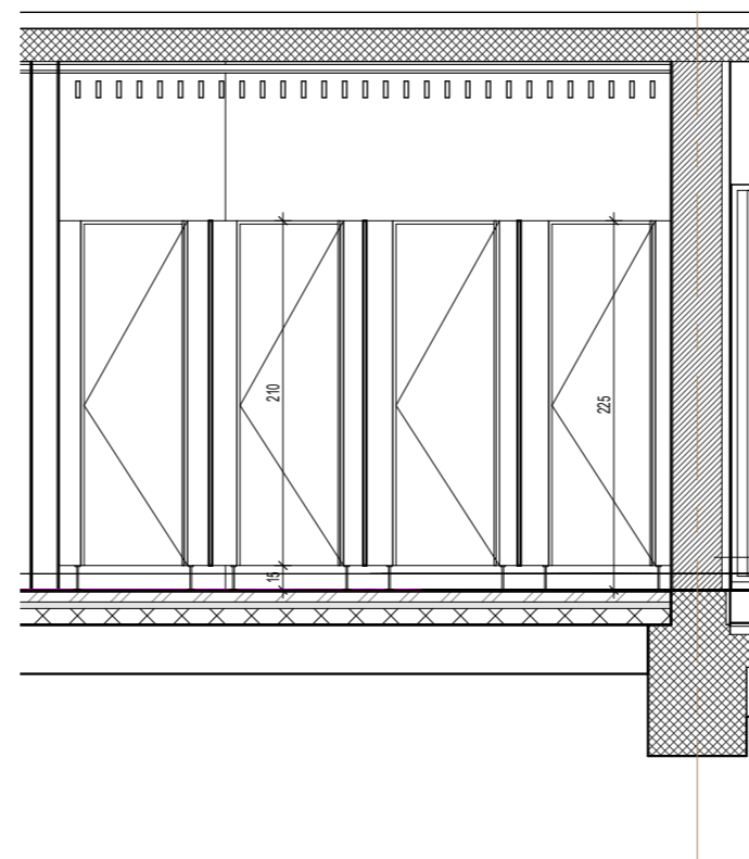
2 Presjek HPL H7-a 1:50
