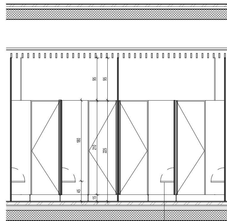
5 Presjek HPL D5-d 1:50
