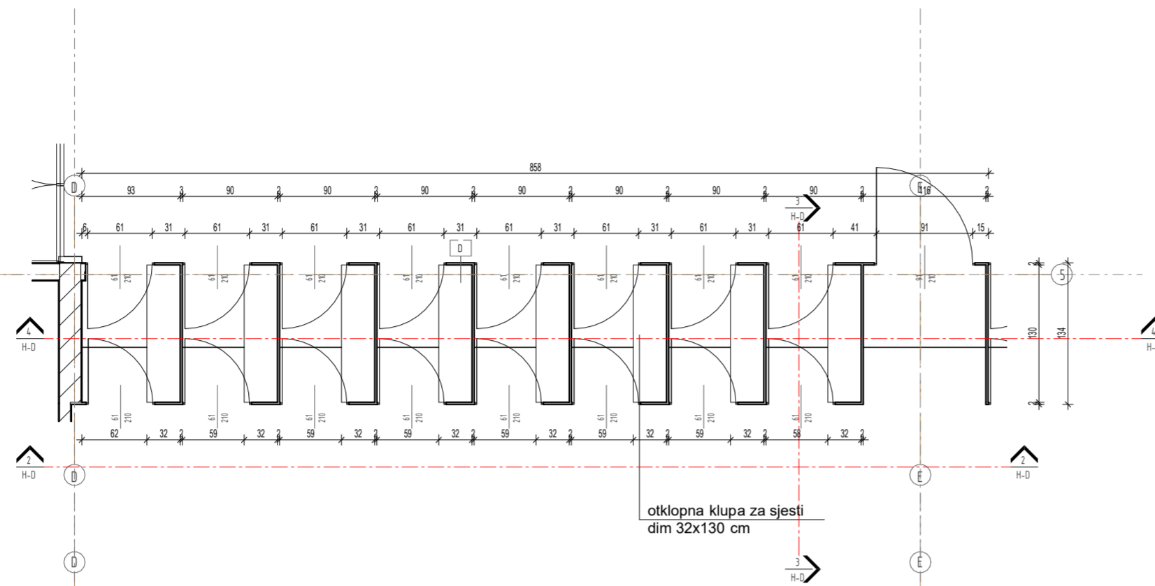
1 Tlocrt HPL D 1:50
