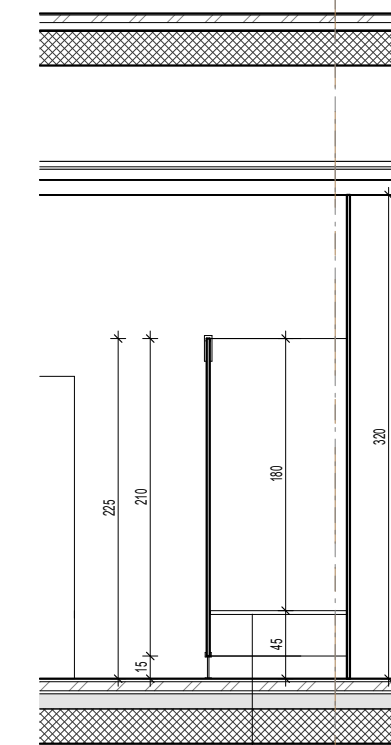
3 Presjek HPL D5-b 1:50
