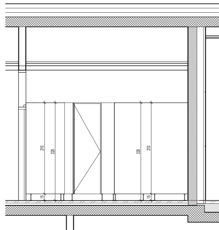
3 Presjek HPL H19 i H20 1:50
