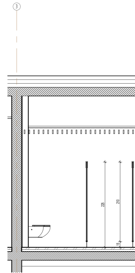
4 Presjek HPL H18, H20 1:50
