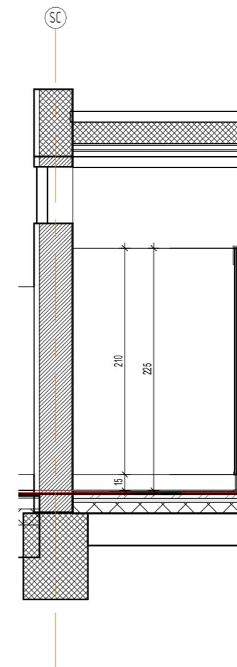
3 Presjek HPL H7-b 1:50
