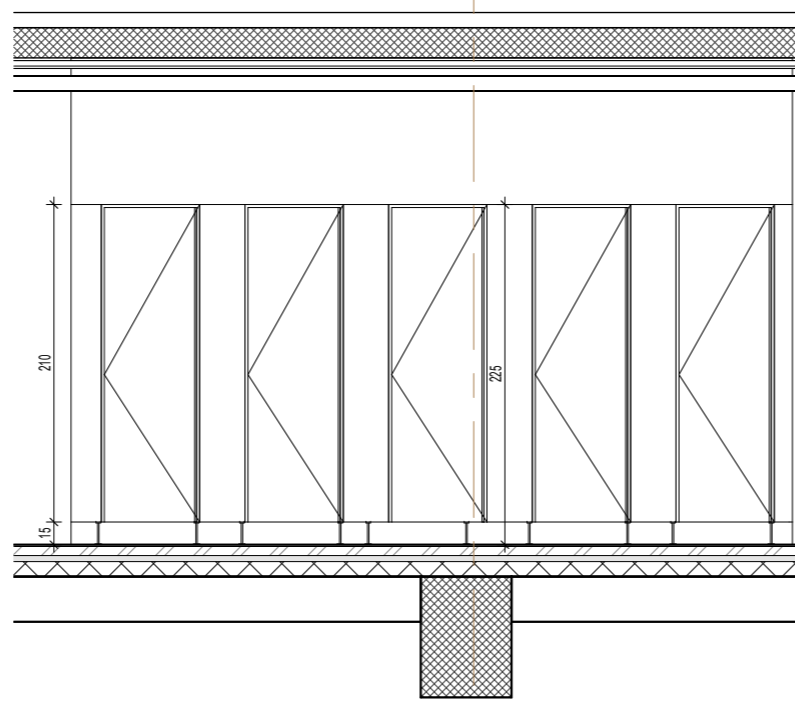
2 1:50 Presjek HPL G-a
