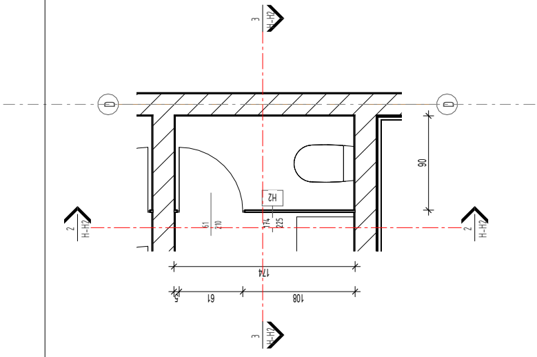
Tlocrt HPL H2 1:50
