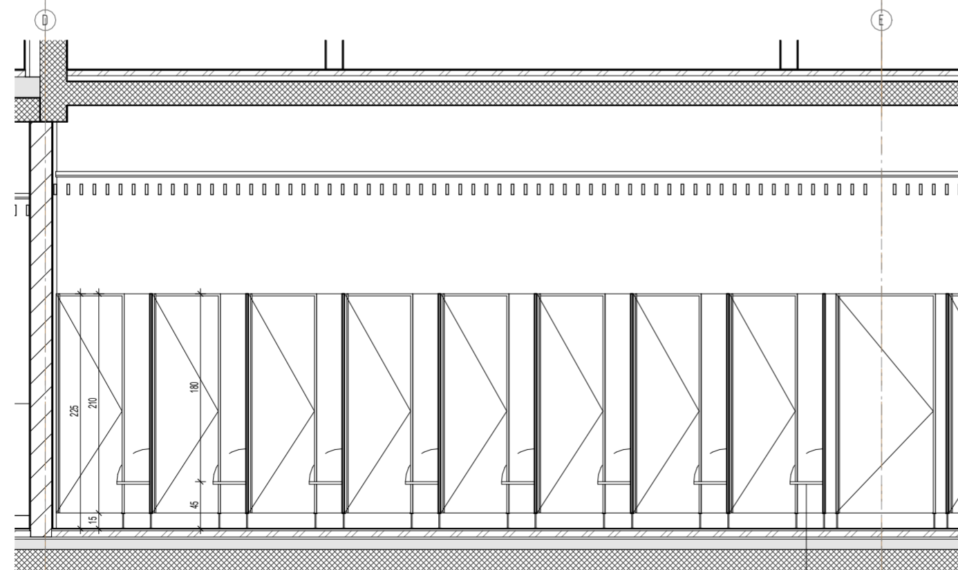
4 Presjek HPL D-c 1:50
