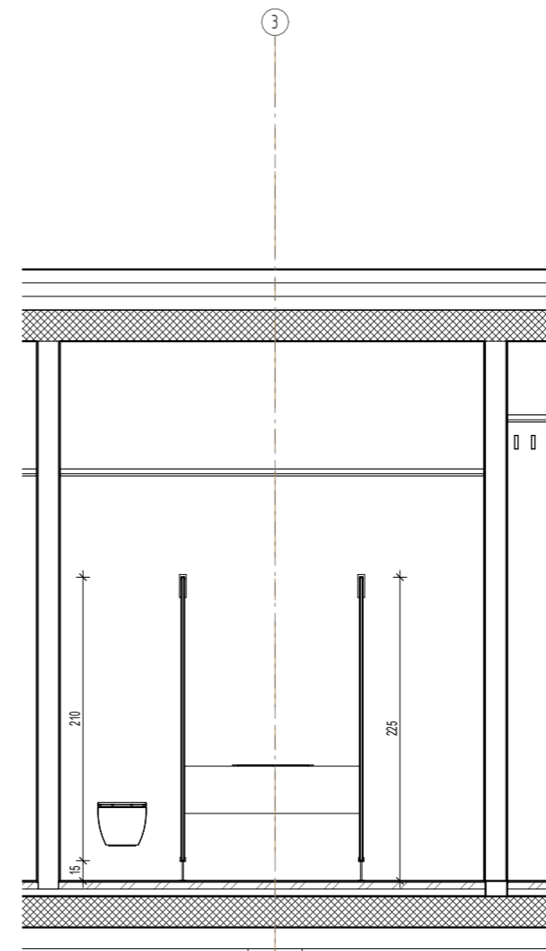
3 Presjek HPL H16-b 1:50
