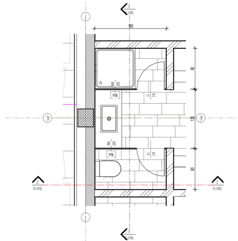
1 Tlocrt HPL H16 1:50
