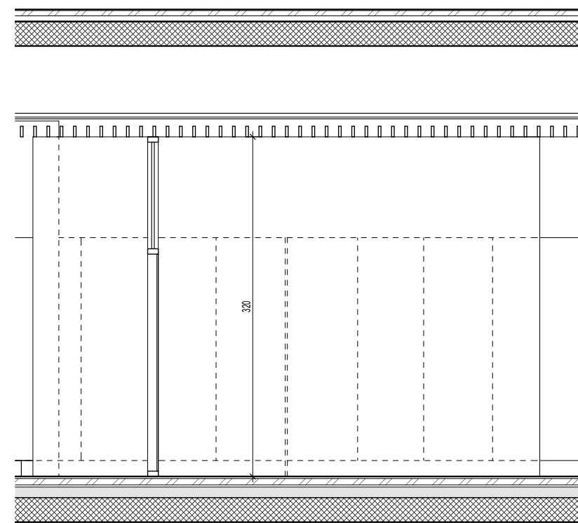
4 Presjek HPL D5-c 1:50
