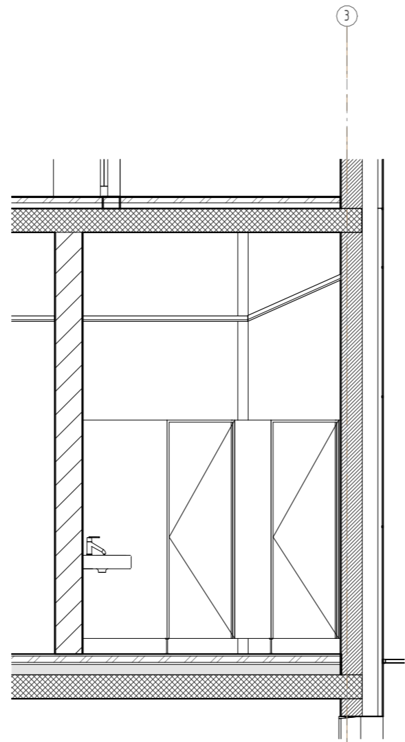
2 Presjek HPL B+B1-a 1:50
