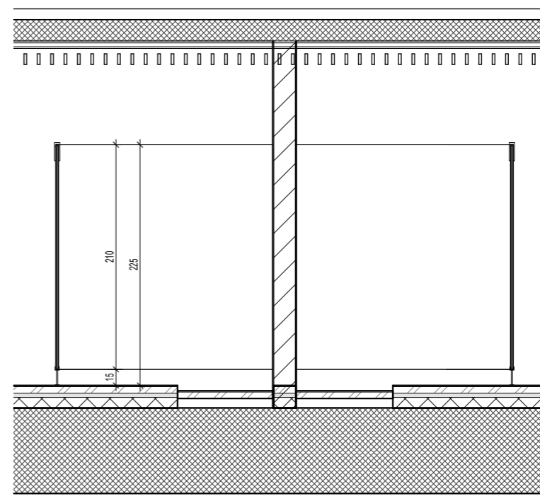
3 1:50 Presjek HPL G-b
