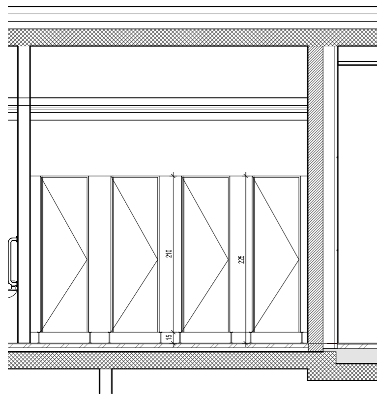
2 Presjek HPL H18-a 1:50
