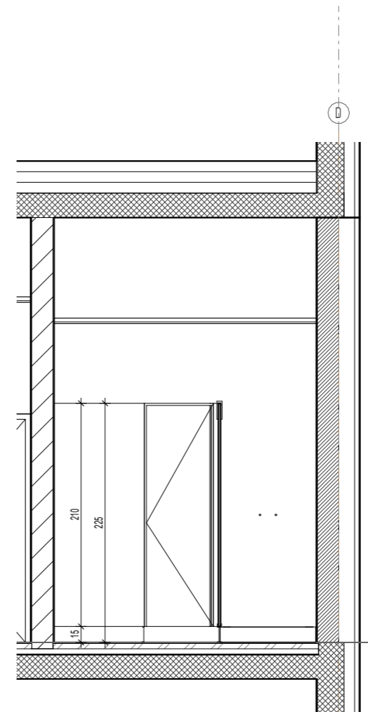
Presjek HPL H8 i H9-a
