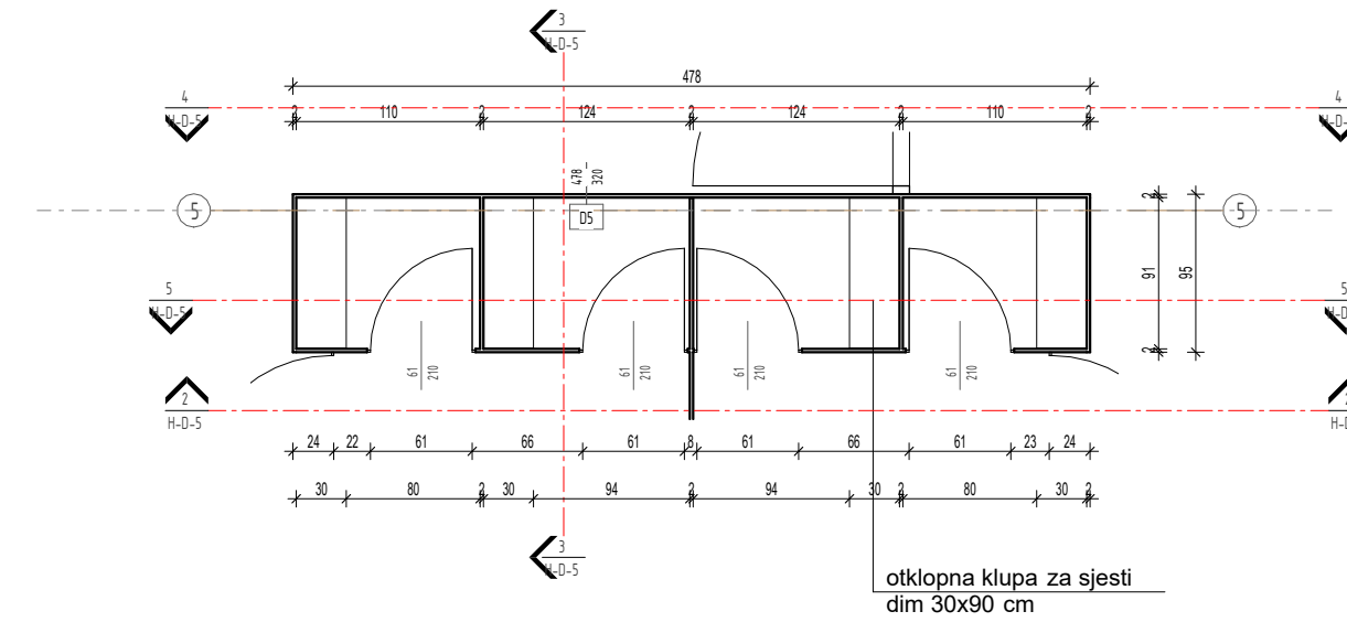
1 Tlocrt HPL D5 1:50
